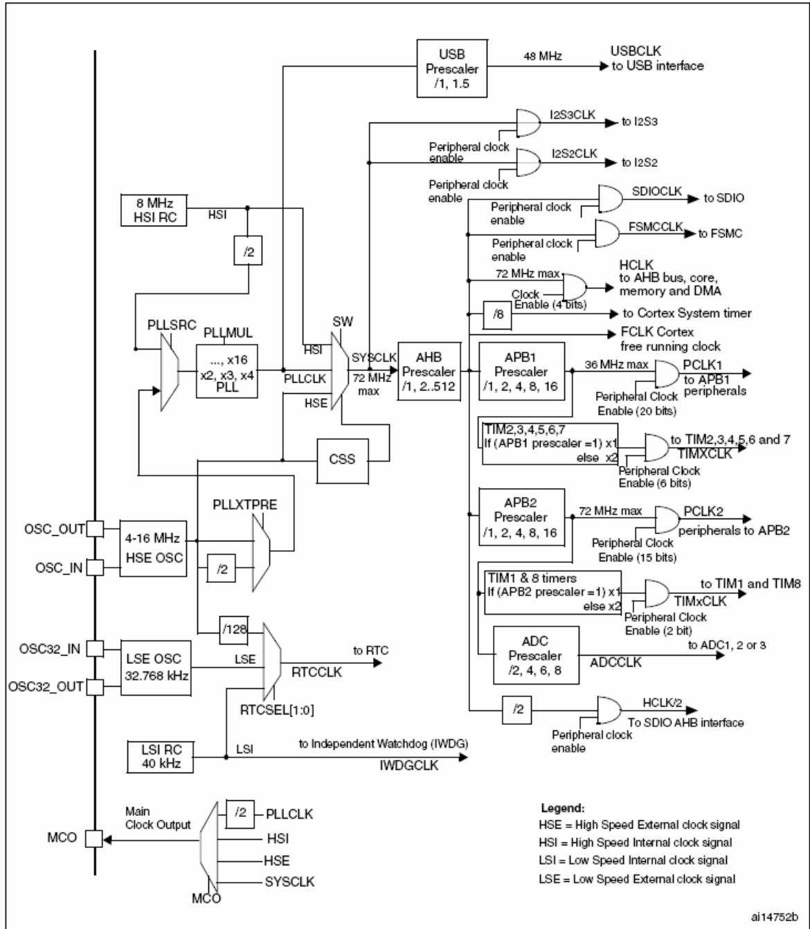
图2 时钟树
