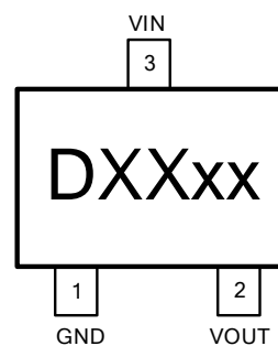
SOT23
