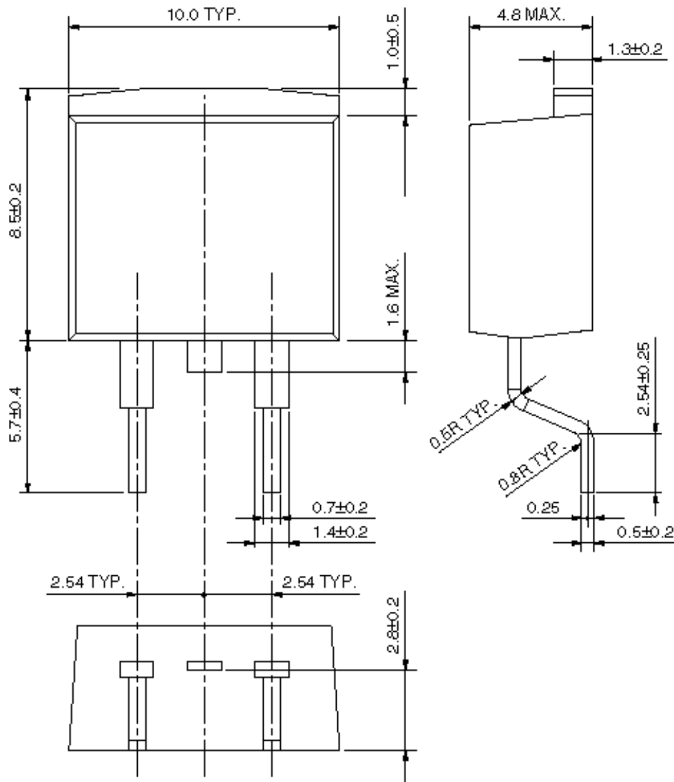
TO-263-2L
